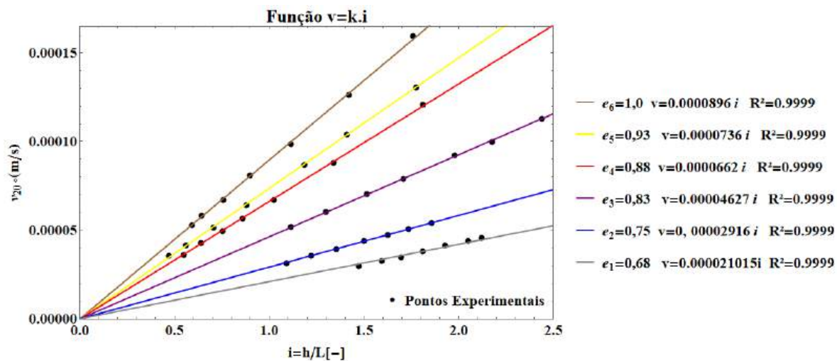
Figura 3. Gráficos de regressão linear obtidos pelos ensaios de permeabilidade do solo em laboratório.
