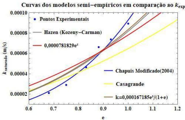
Figura 4. Curvas das expressões semi-empíricas e resultados experimentais obtidos para k .
