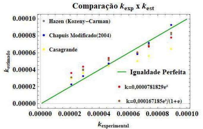
Figura 5. Comparação do k obtido em laboratório e com aplicação das equações semi-empíricas.
