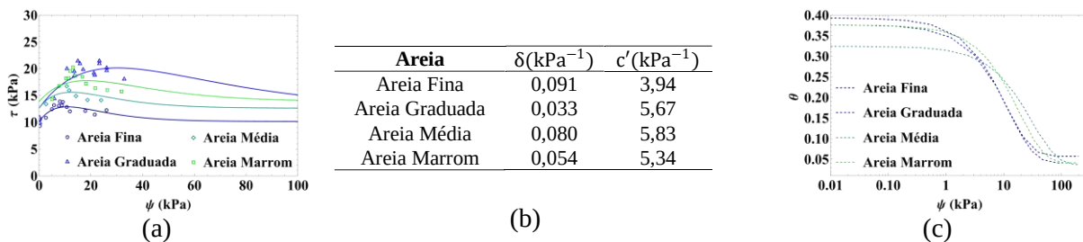
Figura 7. (a) Resistência ao cisalhamento versus sucção para as areias de Frankston obtidas por Donald (1956). (b) Parâmetros do solo ajustados. (c) Curva de Retenção de Água no Solo hipotética para as areias de Frankston com a suposição de que \theta_s é numericamente igual a porosidade \theta_r=0 . (adaptadas de Cavalcante & Mascarenhas (2021)).
