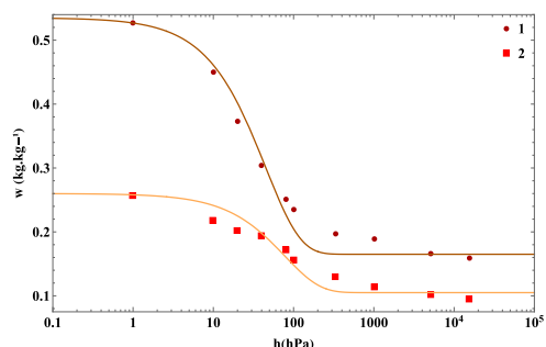
Figura 11. Curva de retenção da água nos solos LVdf e LVec em pontos distintos.
