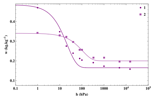
Figura 12. Curva de retenção da água no solo NVec em diferentes posições.
