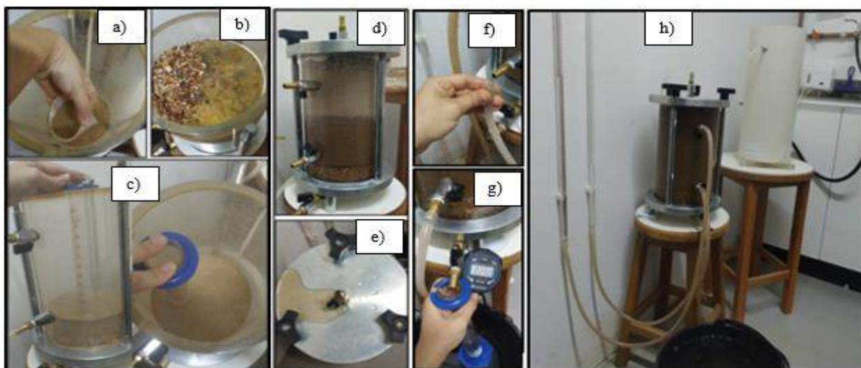
Figura 1. Procedimento do ensaio de permeabilidade.
